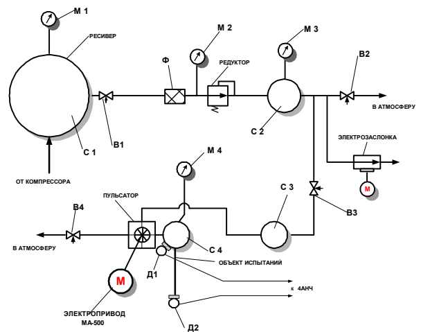
Рис. 1. Пневматическая схема стенда для частотных испытаний зондов при высоком давлении: М1, М2, М3, М4 – манометры; В1, В2, В3, В4 – вентили; С1, С2, С3, С4 – емкости; Ф – фильтр воздушный; Д1, Д2 – датчики пульсаций давления
