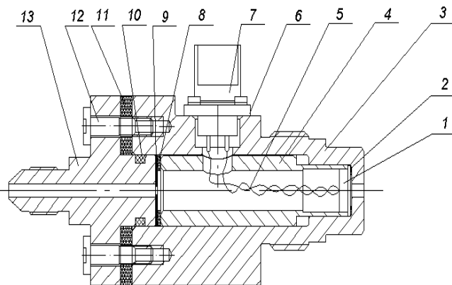
Рис.4. Герметичный корпус с установленным датчиком ДМИ-0.6-1: 1 - датчик ДМИ-0,6-1; 2 - прокладка уплотнительная; 3 - корпус; 4 - прокладка; 5 - провод соединительный; 6 - прокладка; 7 - штепсельный разъем; 8 - прокладка; 9 - дроссельная шайба; 10 - кольцо уплотнительное; 11 - прокладка; 12 - винт; 13 - крышка со штуцером для подвода стационарной составляющей давления
